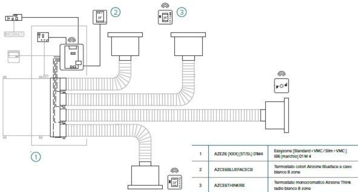
Schema elettrico della installazione
