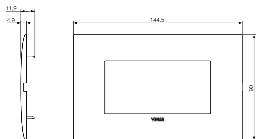
19954... - Placca 4 moduli
