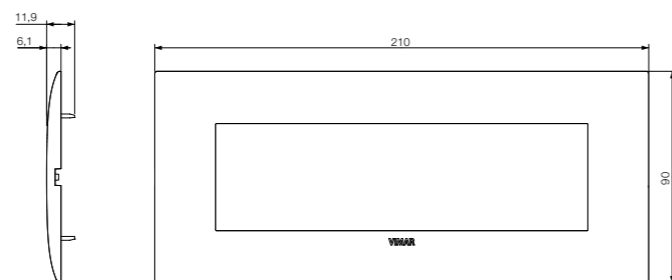
19957... - Placca 7 moduli
