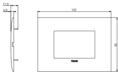
19953... - Placca 3 moduli
